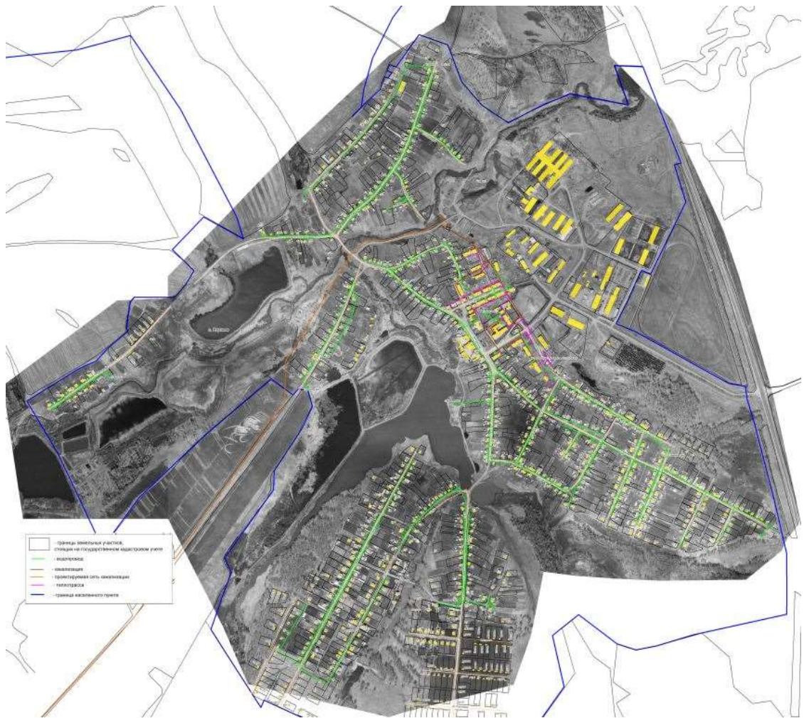
Рис. 3 Существующая зона действия котельной с. Ягуново
