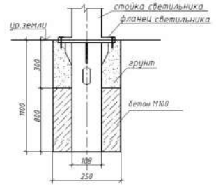
Бетонирование фундамента торшерной стойки
