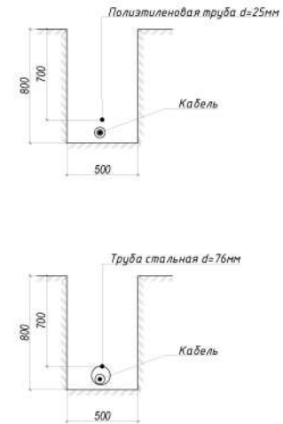
Схема траншеи для прокладки кабеля
